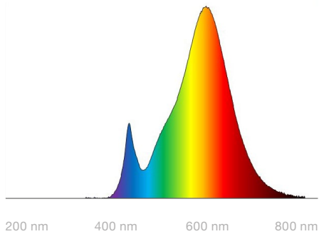
Farbtemperatur 2.700 K
